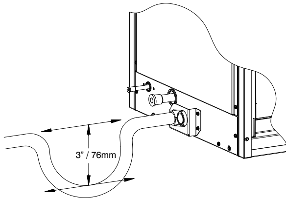
Fig. 8 – Condensate Trap
